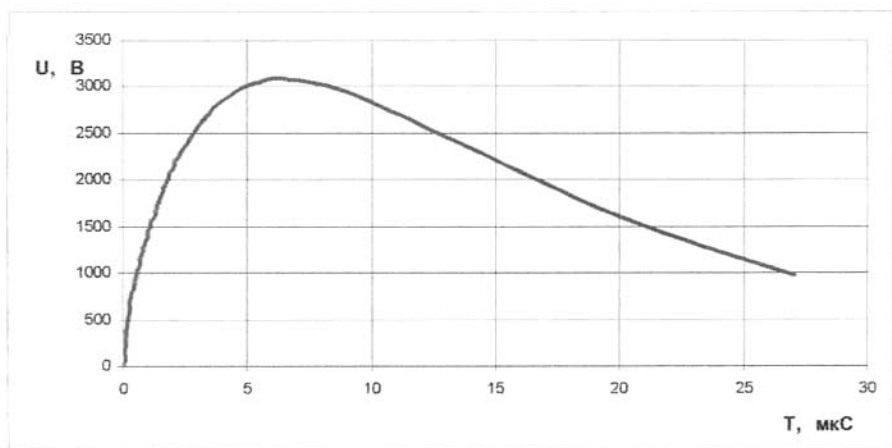
Рис.4а. Типовая осциллограмма воздействующего импульса напряжения.
