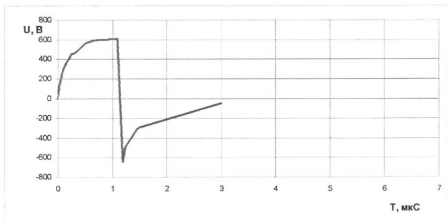
Рис. 4б. Осциллограмма напряжения на выходе ЗАФУ
